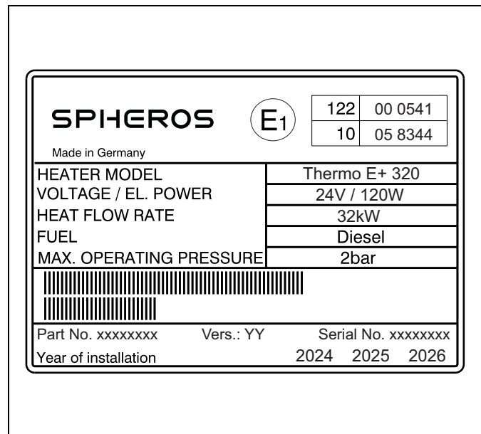
Рисунок 7: Табличка обозначения типа (пример)
